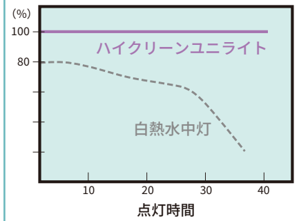
点灯時間による光力変化曲線
